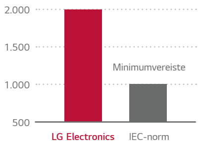
Uren Vocht-warmte-test
